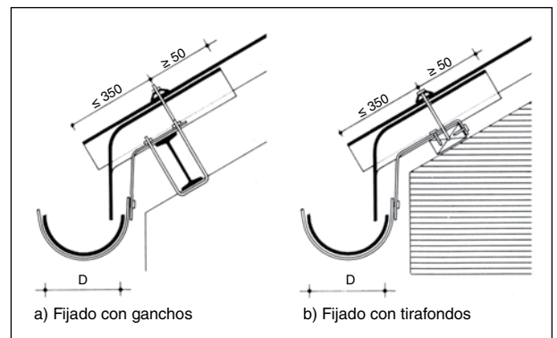
Figura 7. Detalle de la colocación de canalón de fibrocemento.
